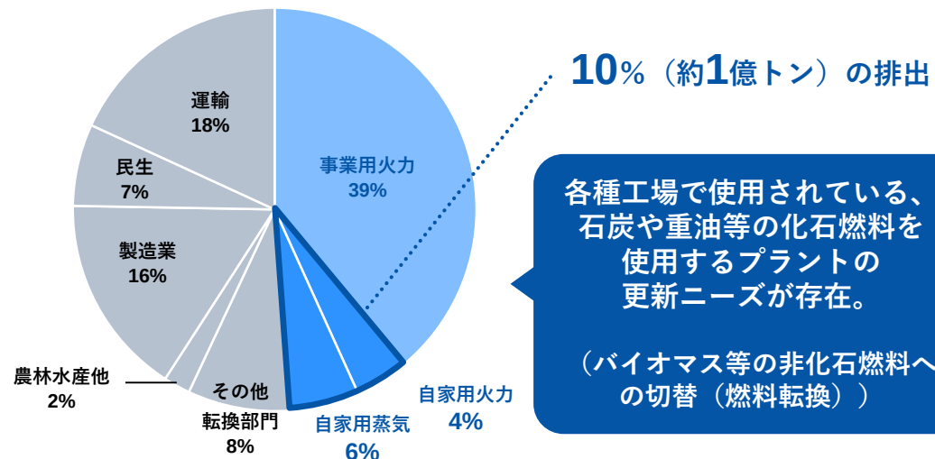
日本のエネルギー起源二酸化炭素排出量※ 4
